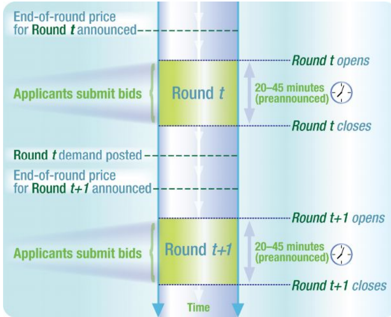
الشكل ٤-٣ - تسلسل الأحداث خلال مزاد التوقيت الصاعد.
