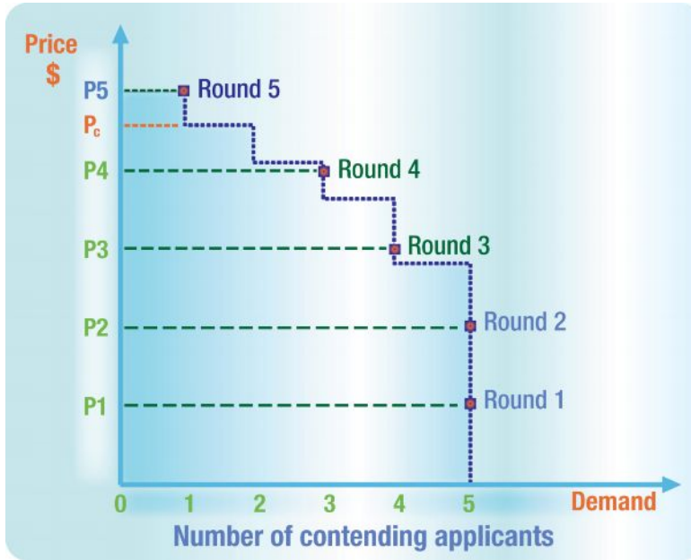
الشكل ٤-٤ - مثال لمزاد ذي خمسة طلبات متنافسة تبادلياً.
