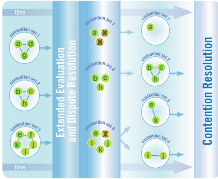
الشكل ٢-٤ - لا يمكن بدء حل التنافس على السلسلة حتى ينهي جميع مقدمي الطلبات داخل إحدى مجموعات التنافس جميع المراحل السابقة المعمول بها.
