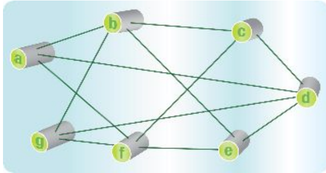
الشكل ٤-١- يمثل هذا الرسم التوضيحي مجموعة تنافس واحدة تعرض كلاً من السلاسل المتنافسة بشكل مباشر والسلاسل المتنافسة بشكل غير مباشر.
